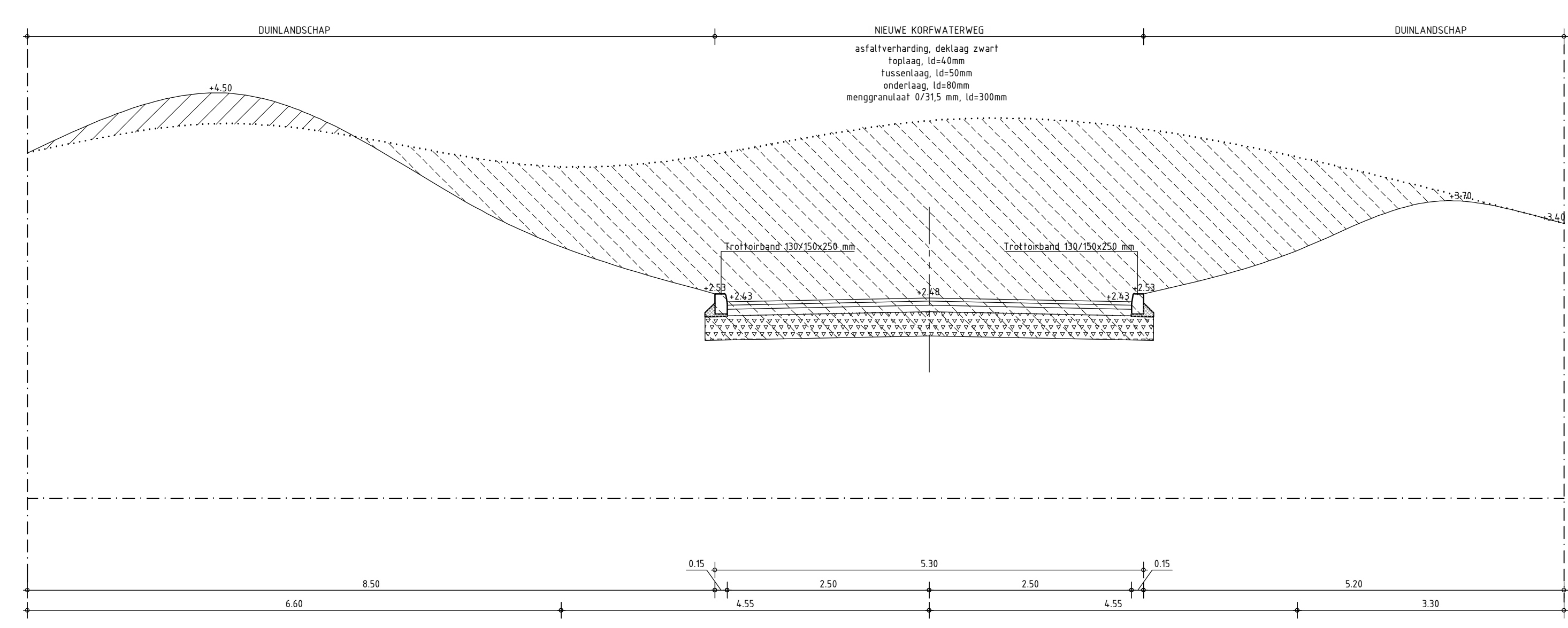
DOORSNEDE F-F 'DWARSDOORSNEDE KORFWATERWEG' SCHAAL 1:50
